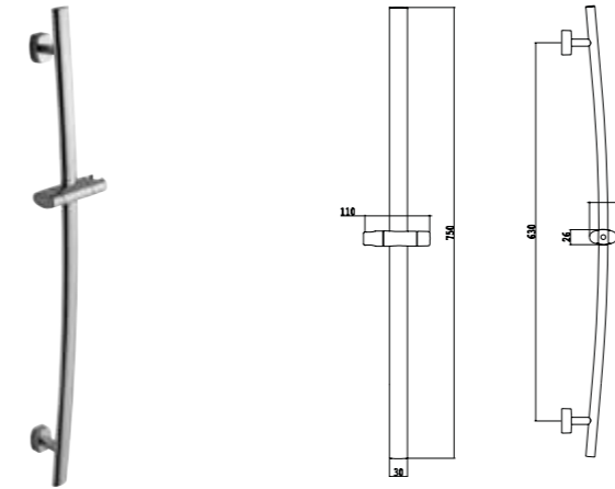
Asta doccia con cursore orientabile L. 750 mm Sliding rail with adjustable shower holder L. 750 mm
