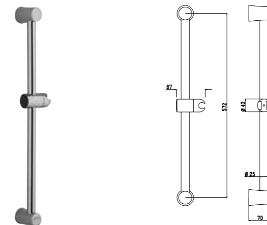
Asta doccia con cursore orientabile L. 600 mm Sliding rail with adjustable shower holder L. 600 mm
