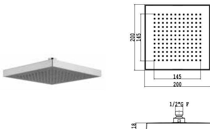
Soffione a pioggia 200x200 mm Rainfall shower head 200x200 mm
