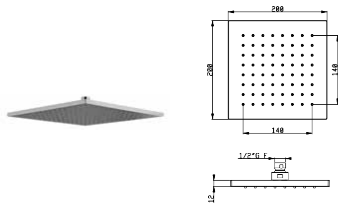
Soffione a pioggia 200x200 // h.12 mm Rainfall shower head 200x200 // h.12 mm
